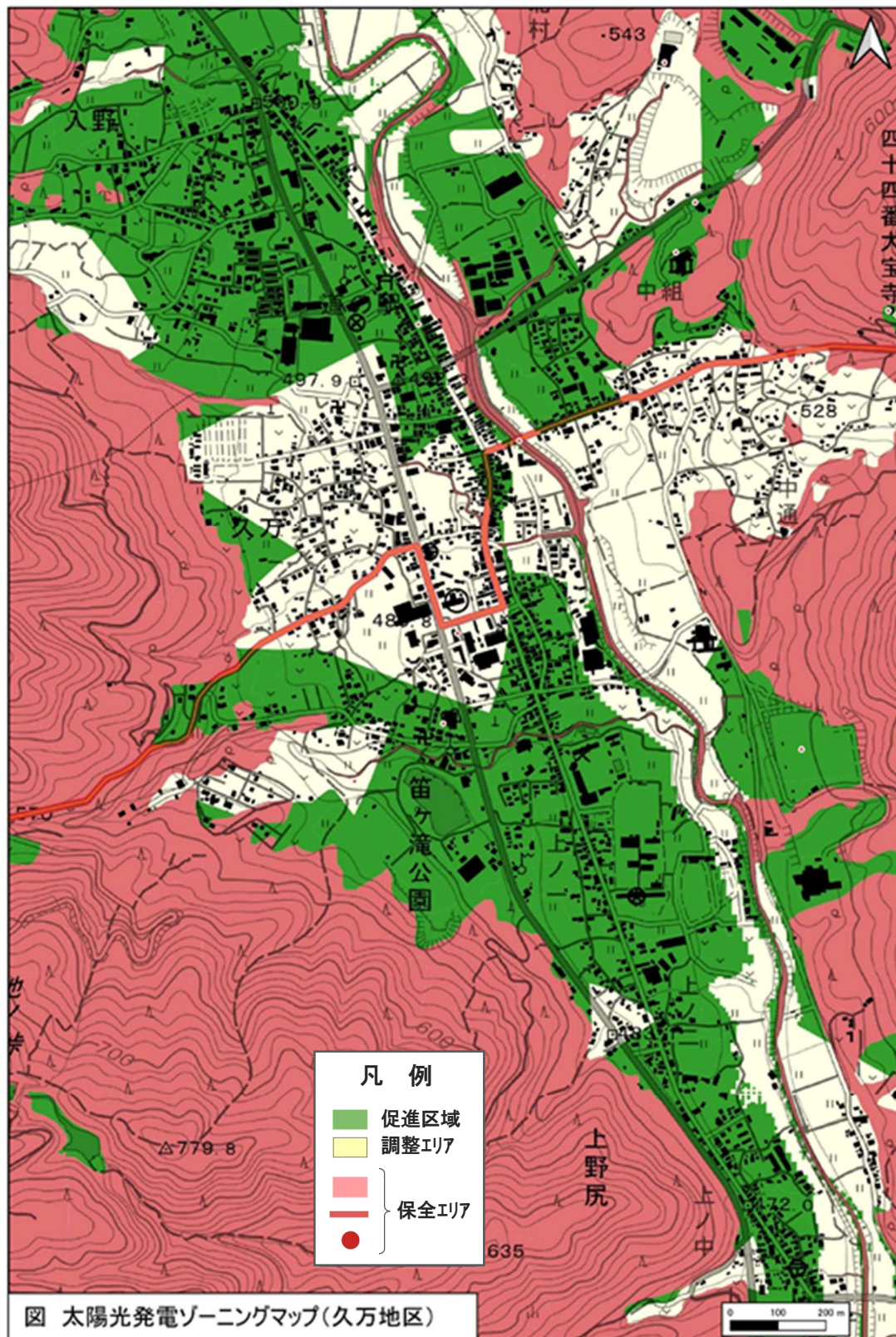
図 1-2 促進区域等ゾーニングマップ（太陽光：久万地区）
