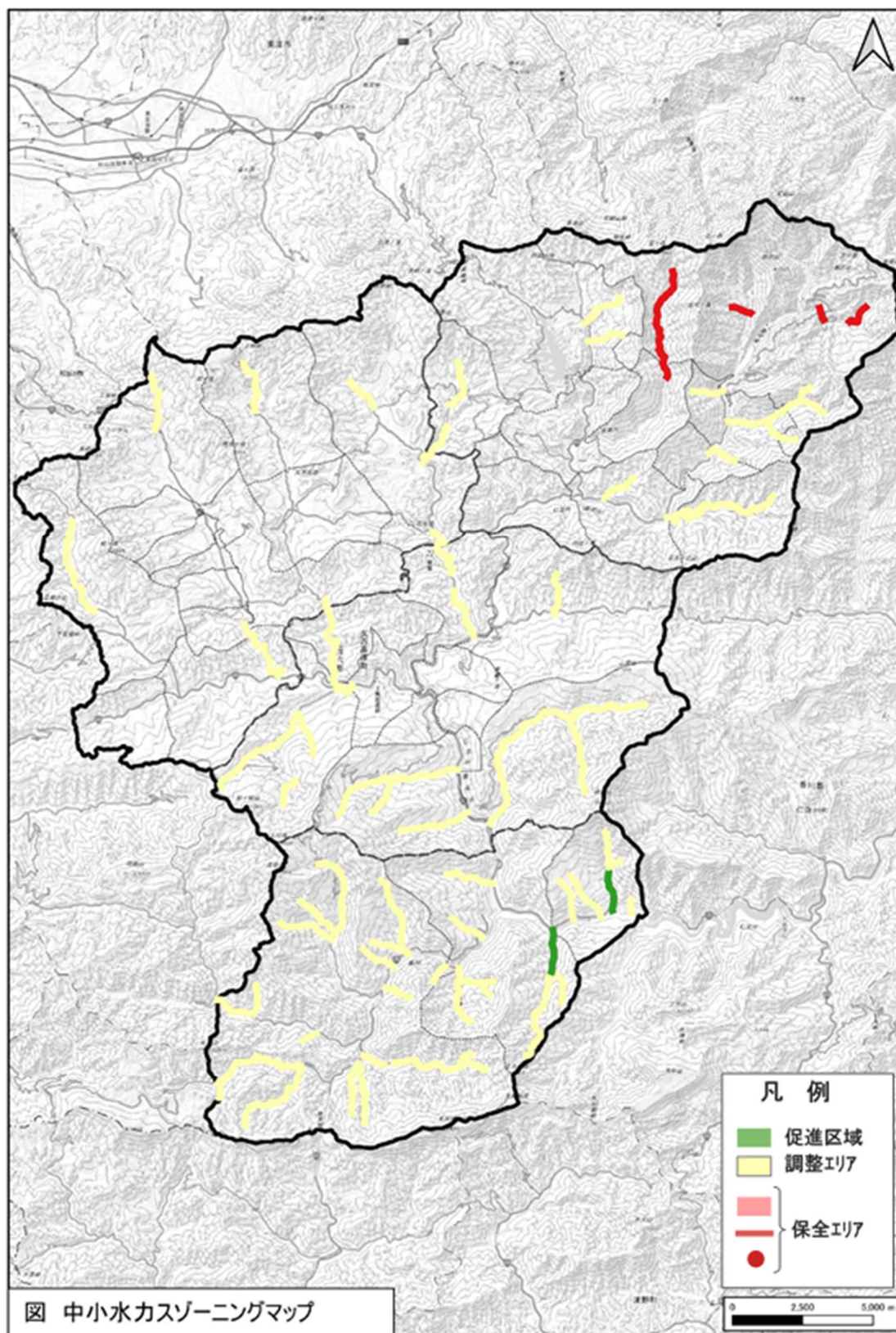
図 4 促進区域等ゾーニングマップ（中小水力）
