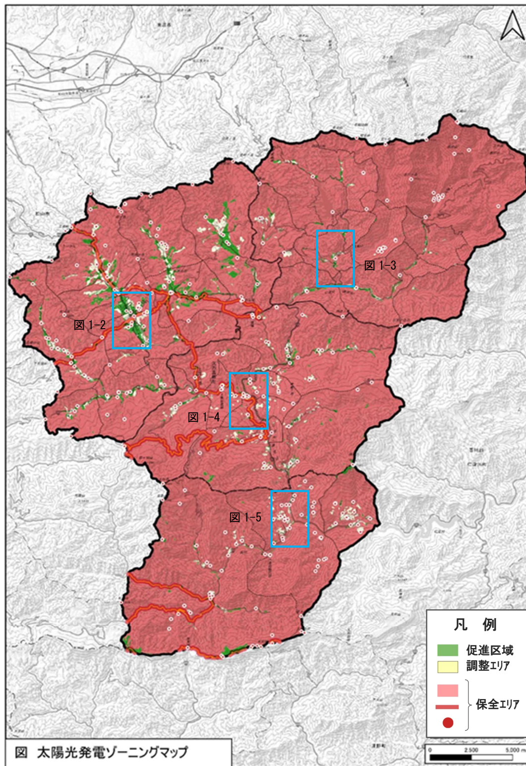
図 1 促進区域等ゾーニングマップ（太陽光）
