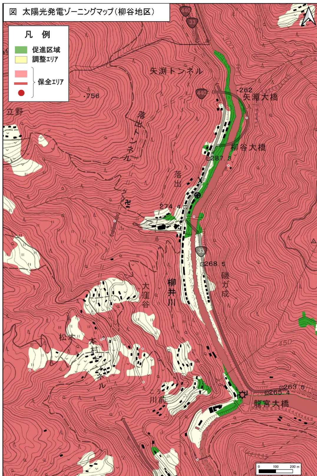
図 1-5 促進区域等ゾーニングマップ(太陽光：柳谷地区)
