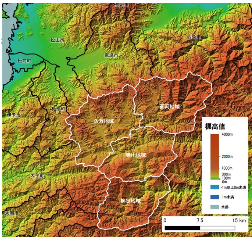
図 2 色別標高図
