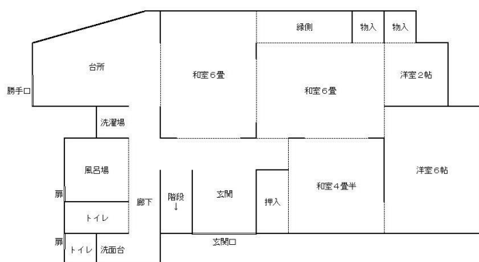
1階
