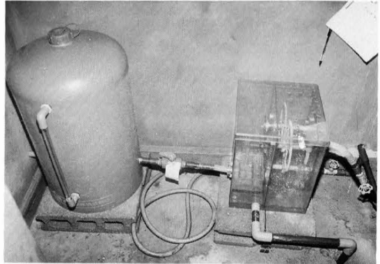
NI 水車型滅菌装置
