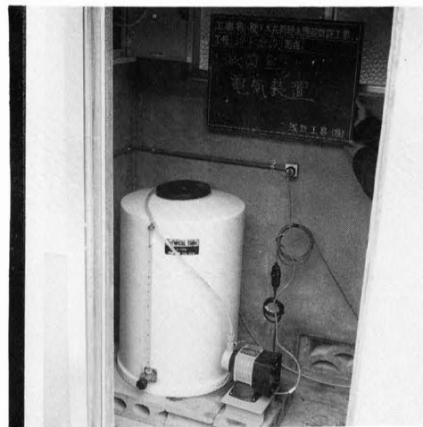
パルス受信方式SP-1P-1型 流量比例式滅菌装置
