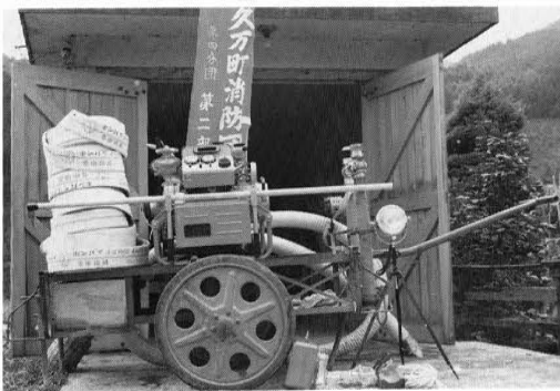
小型動力ポンプ S47年度
